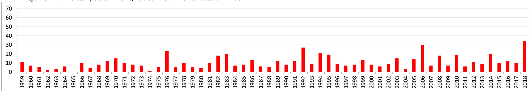
Anzahl Tage Maximum Lufttemperatur > 25 °C, Zeitraum: 01.04.-31.07., Station Emden
