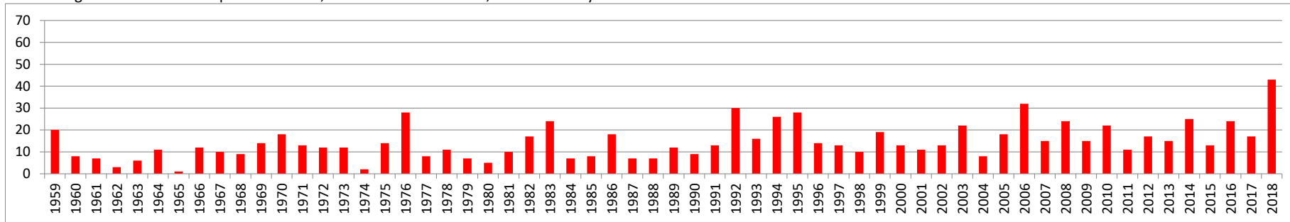
Anzahl Tage Maximum Lufttemperatur > 25 °C, Zeitraum: 01.04.-31.07., Station Friesoythe
