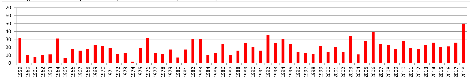
Anzahl Tage Maximum Lufttemperatur > 25 °C, Zeitraum: 01.04.-31.07., Station Göttingen
