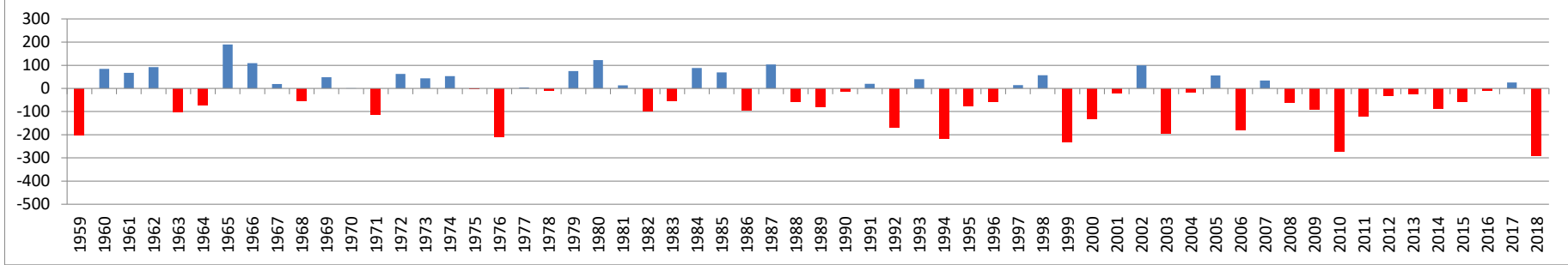
Klimatische Wasserbilanz (mm), Zeitraum: 01.04.-06.08., Station Bremervörde
