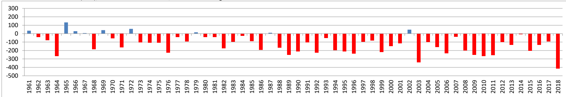
Klimatische Wasserbilanz (mm), Zeitraum: 01.04.-06.08., Station Nienburg
