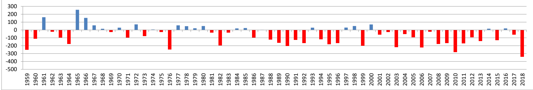
Klimatische Wasserbilanz (mm), Zeitraum: 01.04.-06.08., Station Osnabrück
