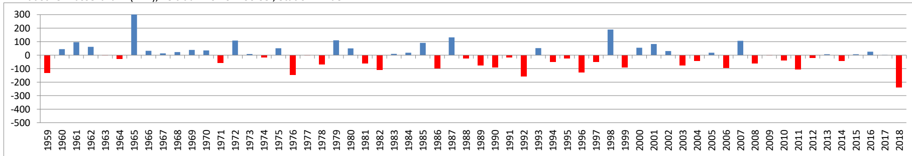
Klimatische Wasserbilanz (mm), Zeitraum: 01.04.-06.08., Station Emden
