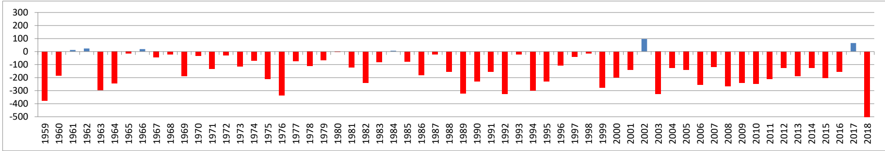
Klimatische Wasserbilanz (mm), Zeitraum: 01.04.-06.08., Station Lüchow
