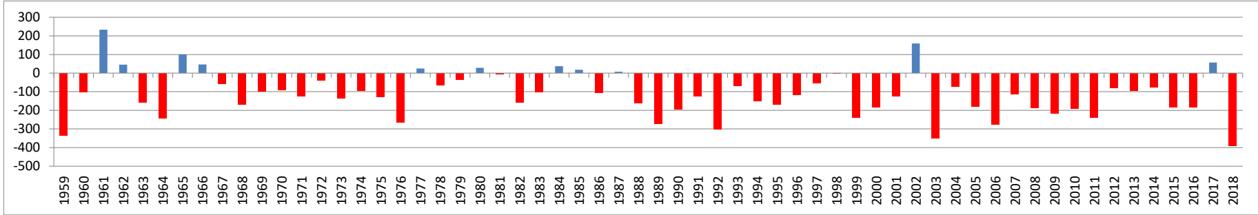
Klimatische Wasserbilanz (mm), Zeitraum: 01.04.-06.08., Station Braunschweig
