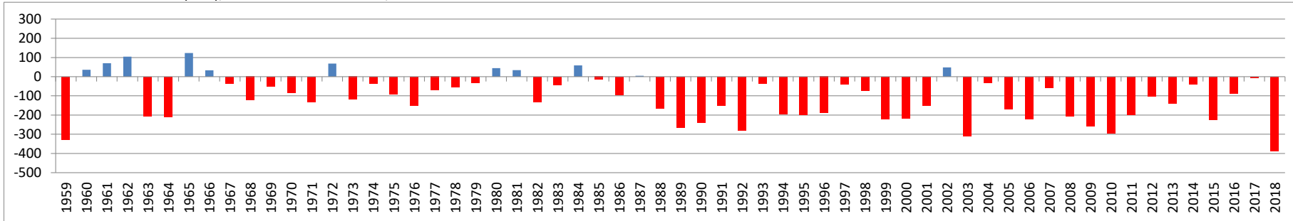
Klimatische Wasserbilanz (mm), Zeitraum: 01.04.-06.08., Station Hannover
