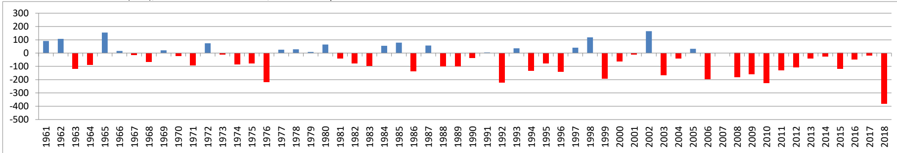
Klimatische Wasserbilanz (mm), Zeitraum: 01.04.-06.08., Station Worswede
