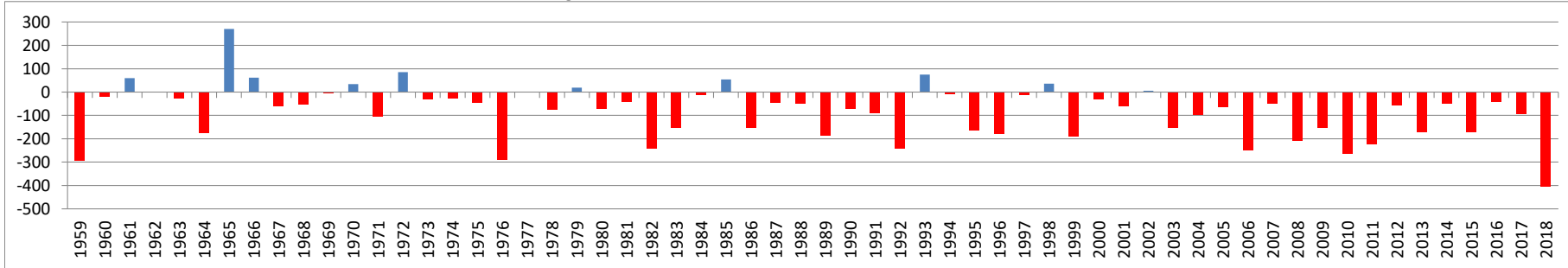
Klimatische Wasserbilanz (mm), Zeitraum: 01.04.-06.08., Station Lingen
