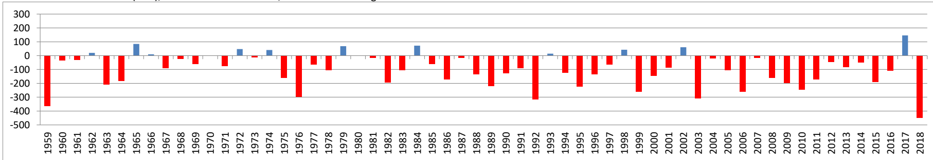
Klimatische Wasserbilanz (mm), Zeitraum: 01.04.-06.08., Station Boizenburg
