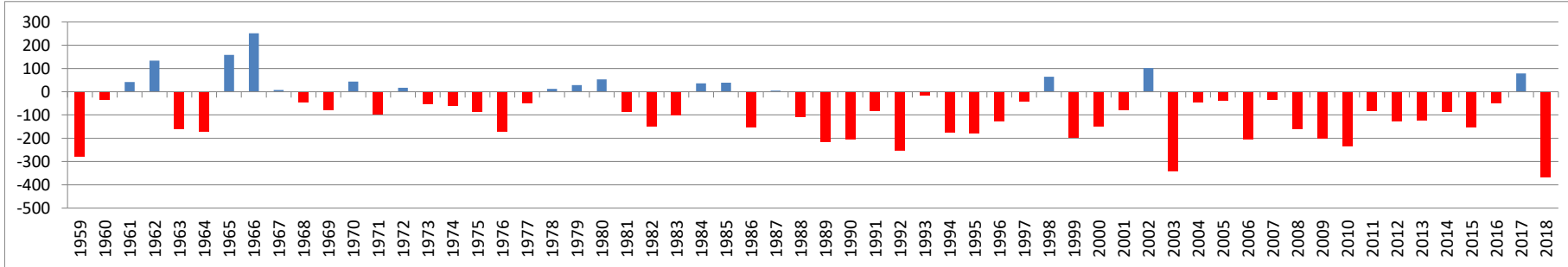
Klimatische Wasserbilanz (mm), Zeitraum: 01.04.-06.08., Station Soltau
