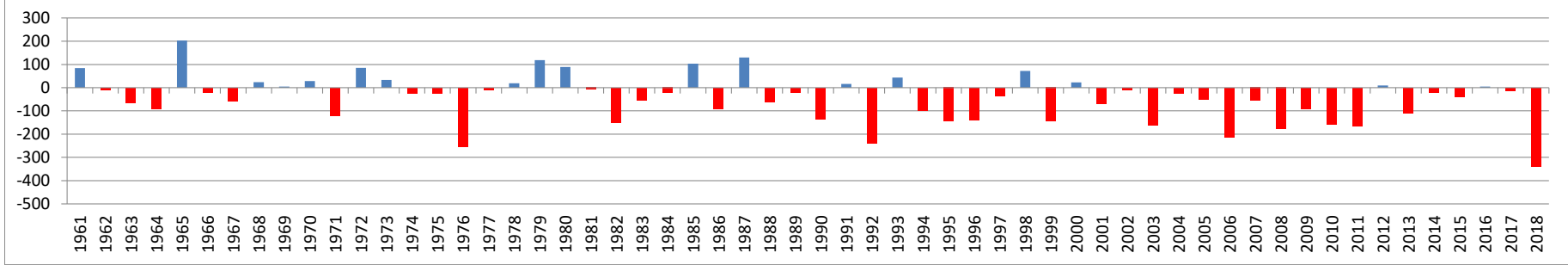
Klimatische Wasserbilanz (mm), Zeitraum: 01.04.-06.08., Station Dörpen
