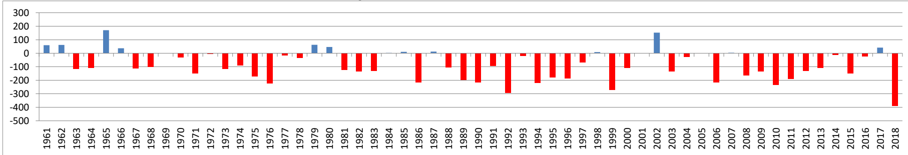
Klimatische Wasserbilanz (mm), Zeitraum: 01.04.-06.08., Station Rotenburg
