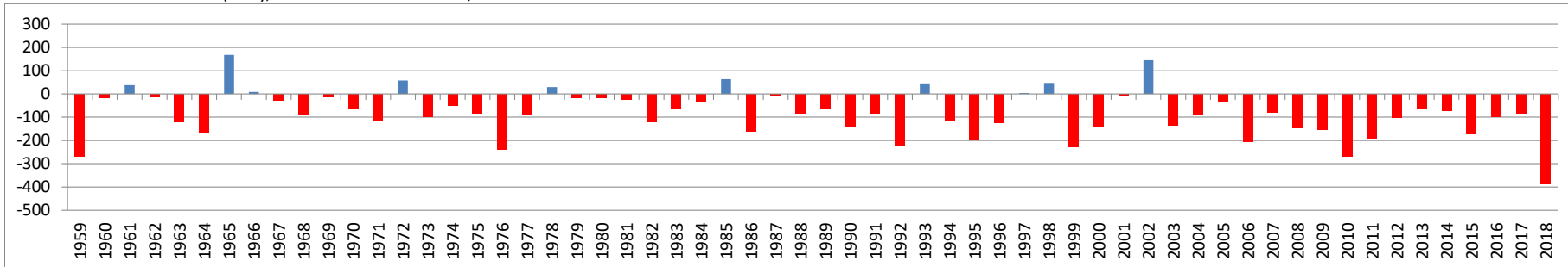
Klimatische Wasserbilanz (mm), Zeitraum: 01.04.-06.08., Station Bremen
