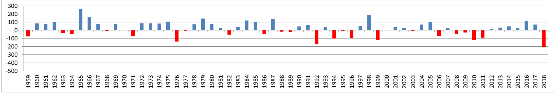
Klimatische Wasserbilanz (mm), Zeitraum: 01.04.-06.08., Station Bremerhaven
