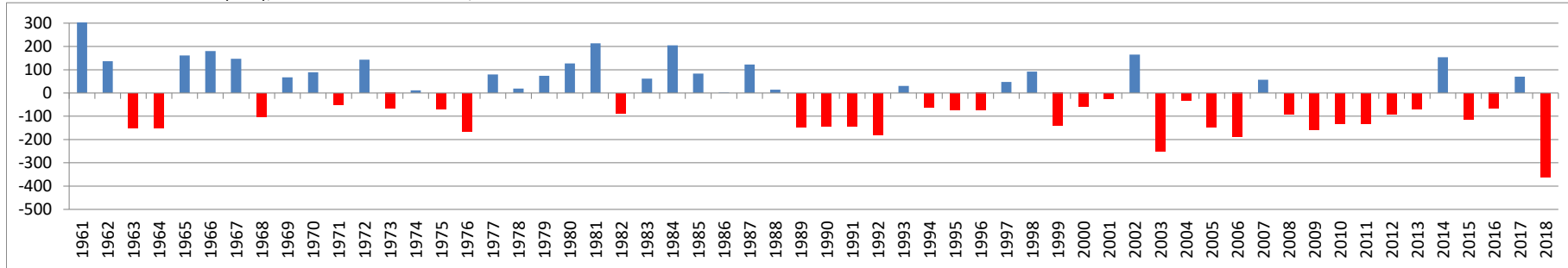
Klimatische Wasserbilanz (mm), Zeitraum: 01.04.-06.08., Station Seesen
